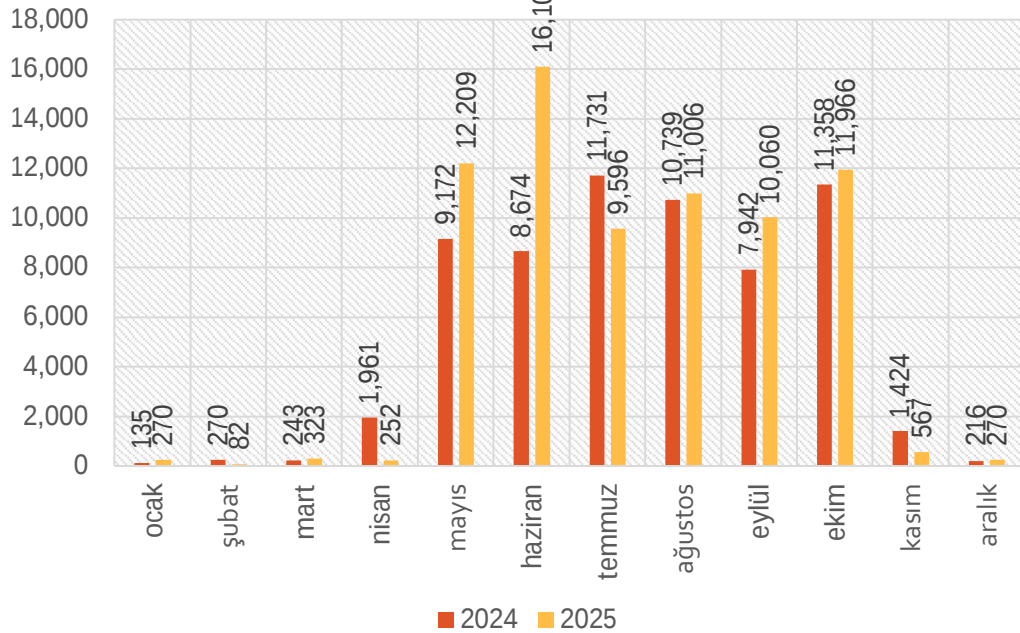
2024-2025 LNG TÜKETİMİ (KG) / AY
